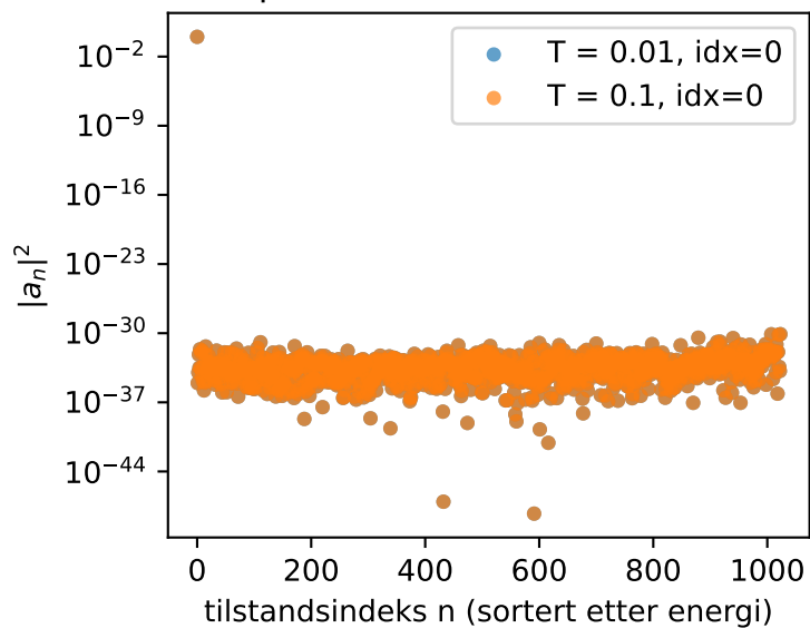
Amplituder vs indeks (tid idx=0)
