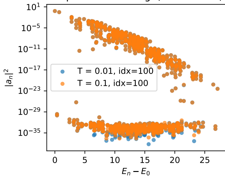
Amplituder vs energi (tid idx=100)
