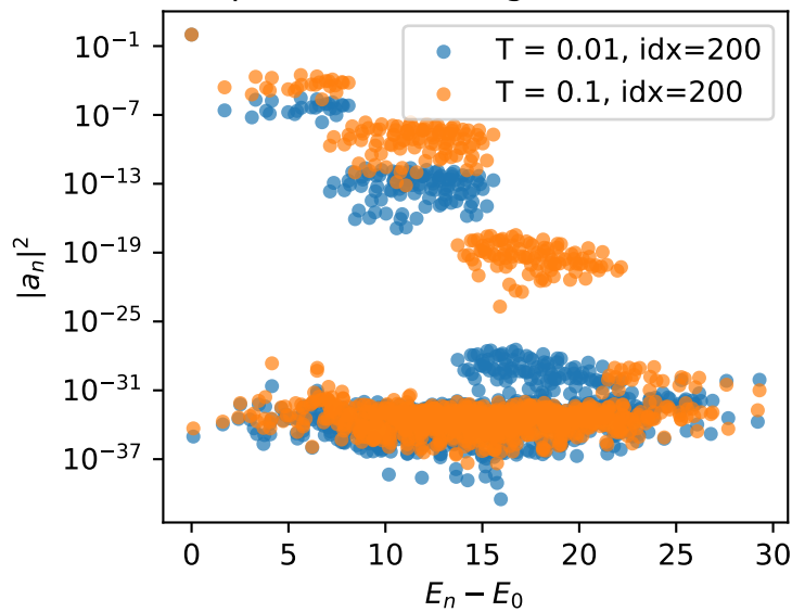
Amplituder vs energi (tid idx=200)
