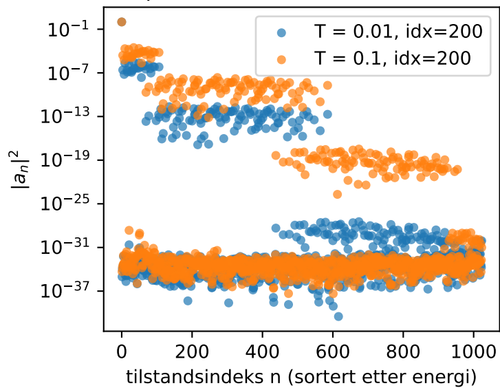
Amplituder vs indeks (tid idx=200)
