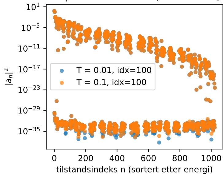
Amplituder vs indeks (tid idx=100)
